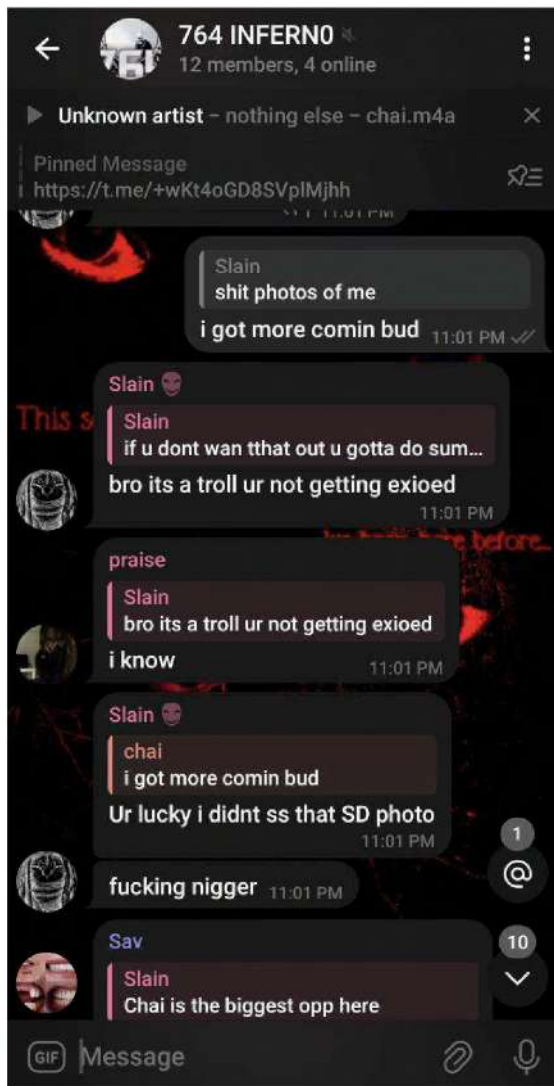
Figur 2: Gruppchatten 764 inferno.
